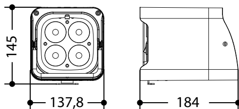
Disegno tecnico
