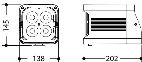
Disegno tecnico
